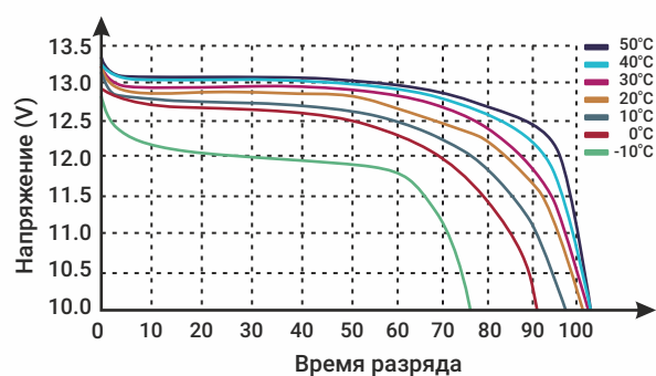
Температура/Время разряда
