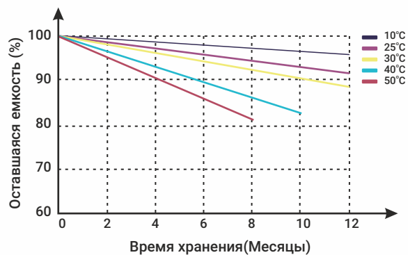
Саморазряд/Температура
